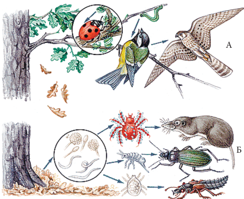
Расми 16. Мисоли занҷири ғизоии рӯйизаминӣ:
